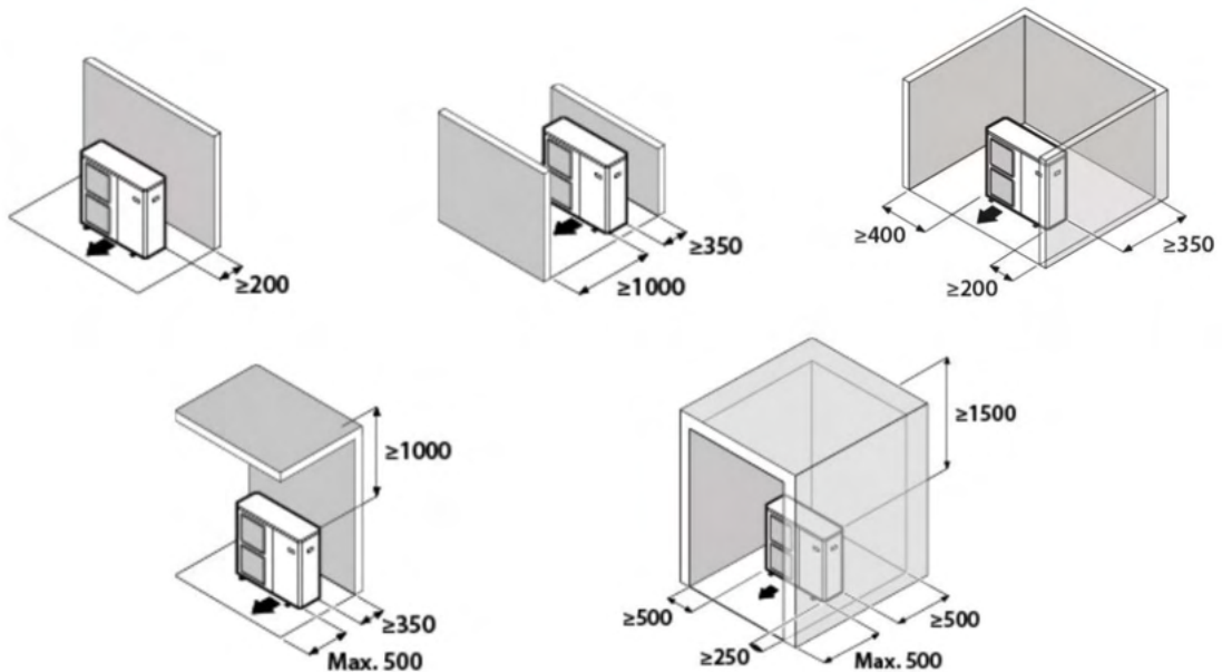
Mindestabstände für den Einbau eines Gerätes (mm).
