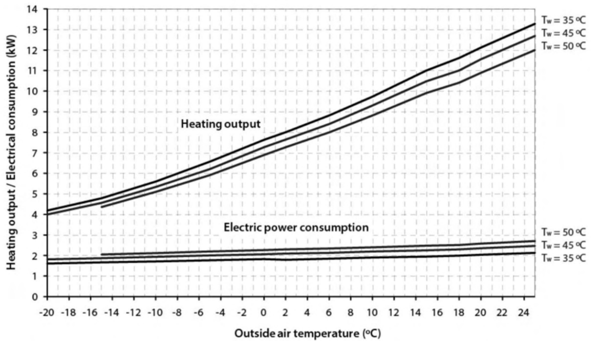
PLW 9 Heizleistung (COP)
