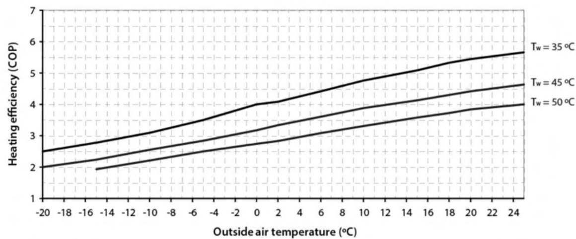
PLW 19 Heizleistung (COP)
