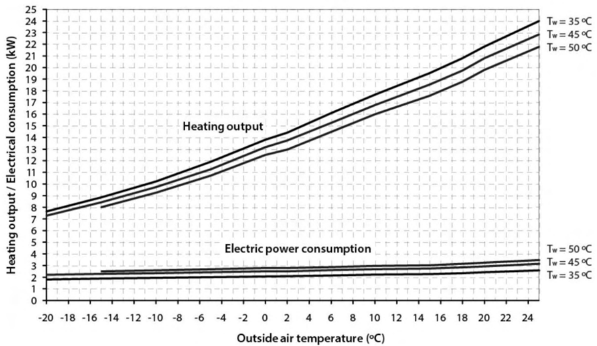
PLW 16 Heizleistung (COP)
