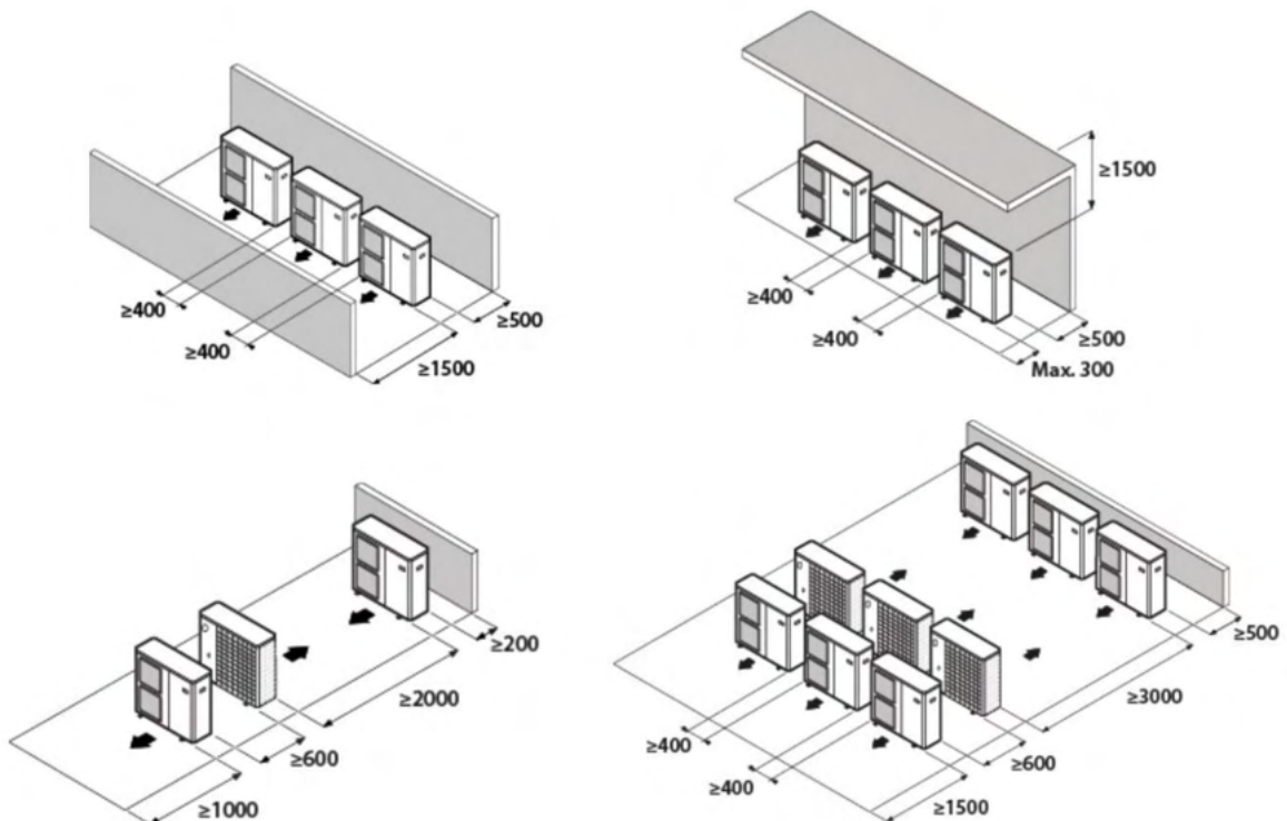
Mindestabstände für die Installation mehrerer Geräte am selben Ort (mm).
