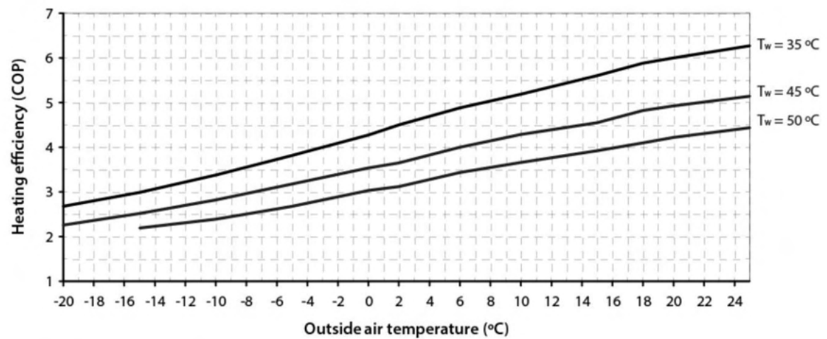
PLW 9 Heizleistung (COP)
