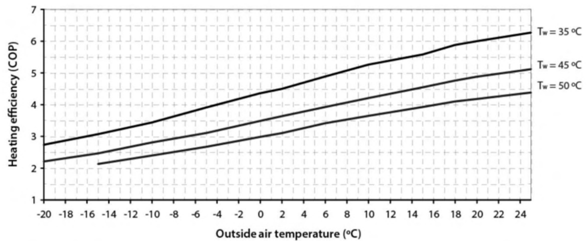
PLW 16 Heizleistung (COP)
