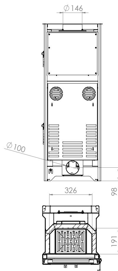
PRZEKRÓJ B-B
