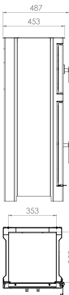
PRZEKRÓJ A-A
