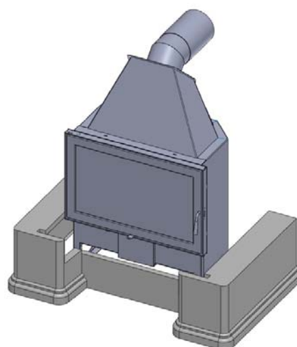
Abbildung 2: Montage der Sockelelemente u. Sockelblende
