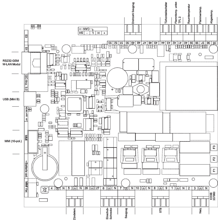
Anschlussplan IO 33.3
