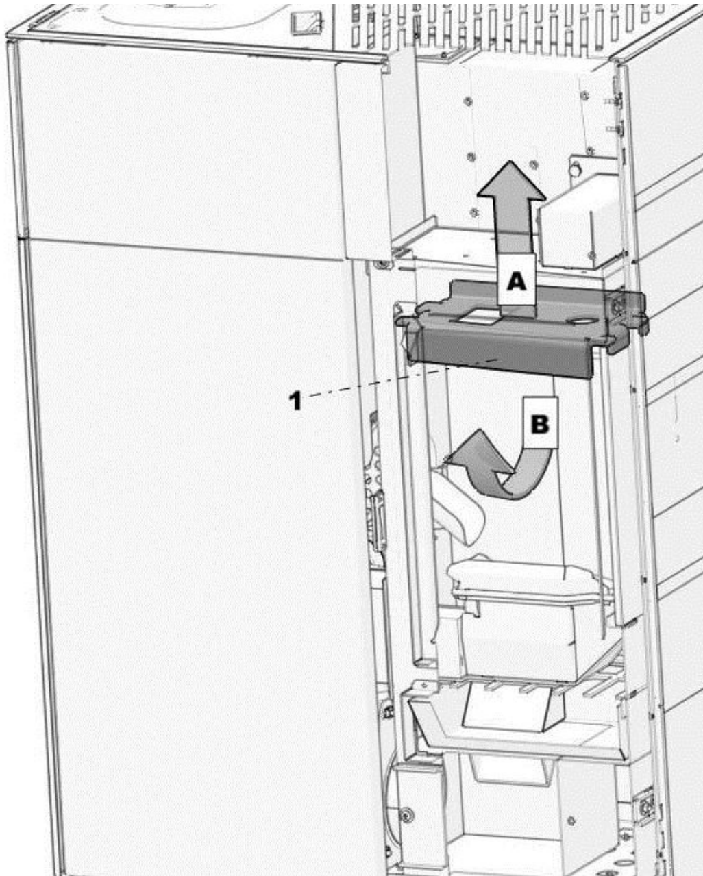
Abbildung 8a: Demontage der Zugumlenkung
