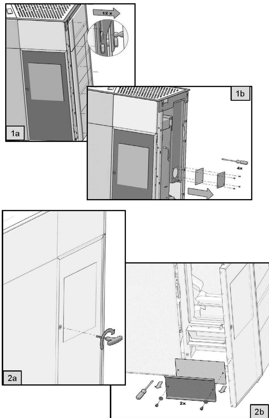
Abbildungen 8b: Demontage der Seitenwand
