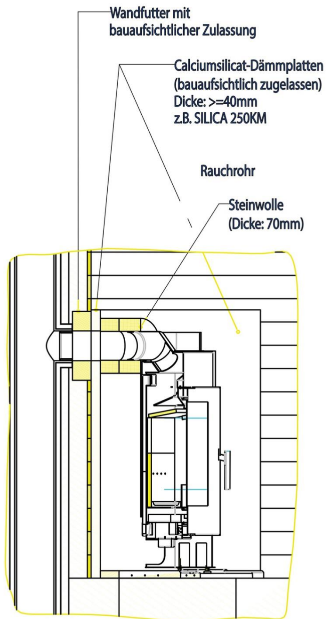
Abbildung 20: Schnittbild Brandschutzvorgaben
