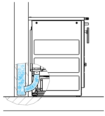
Luftzuleitung von oben Nur mit geprüften Schornsteinsystem
