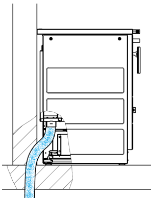
Luftzuleitung von unten max. Schlauchlänge 4m
