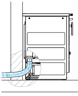
Luftzuleitung von hinten max. Schlauchlänge 4m
