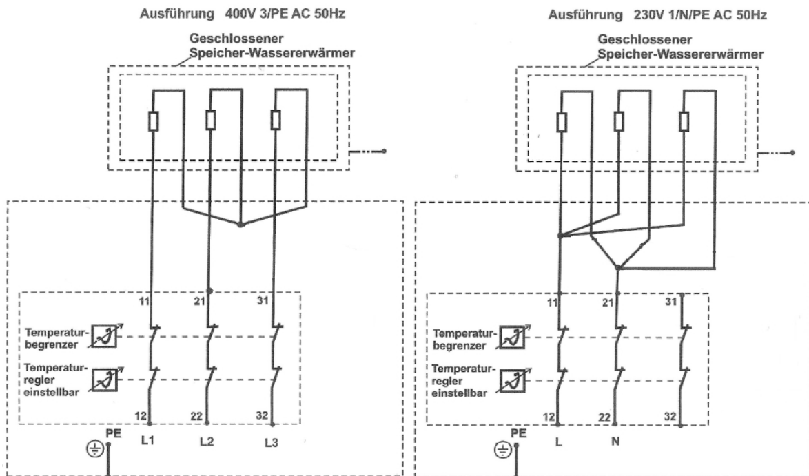
Schaltbild Einschraubheizkörper
